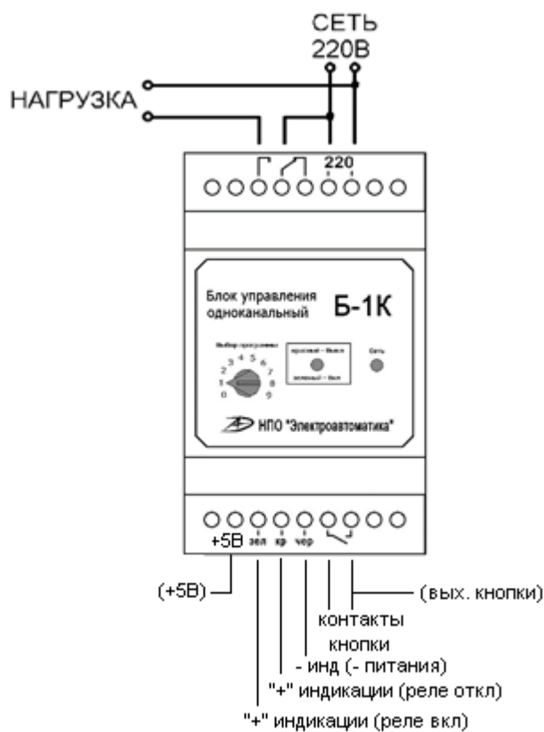
Рис. 2 Подключение устройства
