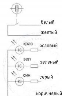
Рис.2 Схема электрическая с общим катодом
