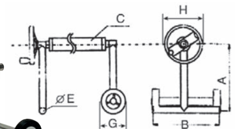
Пример установки суппорта
